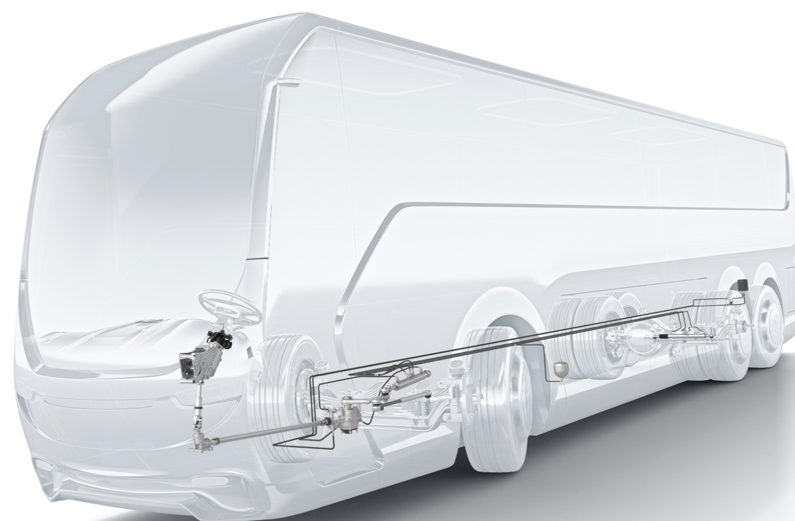
Systemy riadenia zadných náprav pre úžitkové vozidlá
